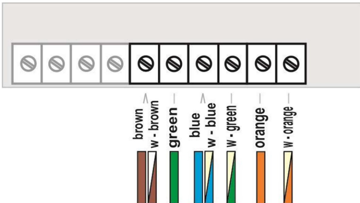
Abbildung 1 Klemmenbelegung PoE
